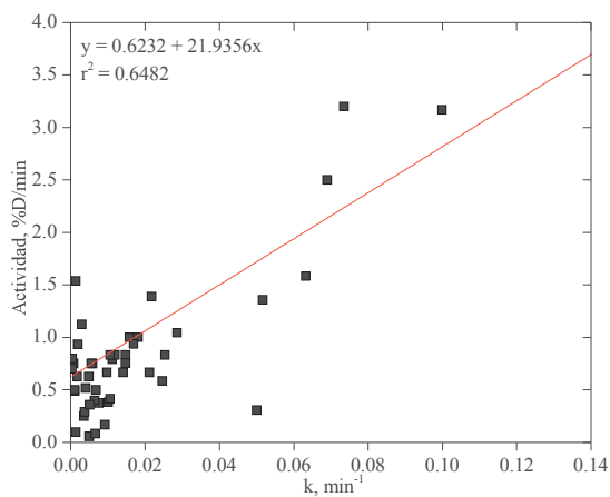
Gráfico 1.1 Actividad vs Constante de rapidez de reacción
