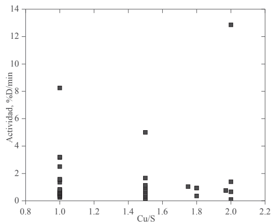
Gráfico 1.2 Actividad vs Relación de Cu/S.
