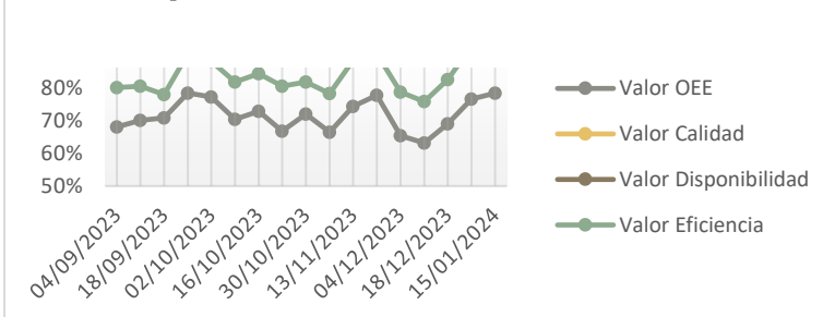
Gráfica 1 Comportamiento semanal de OEE. Extraídos de datos de la industria del caso práctico, 2024
