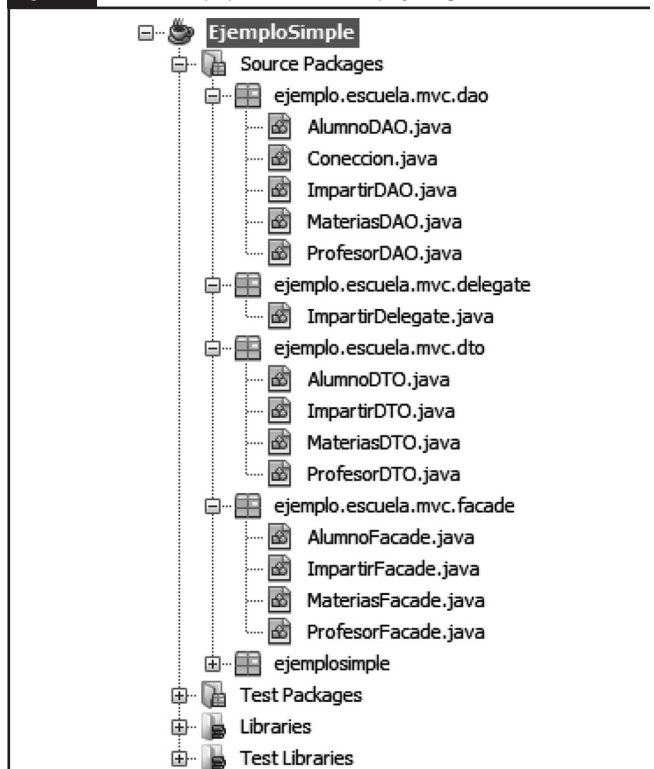
Figura 11. Estructura de paquetes resultante del proyecto generado con GAPRIP MVC.
