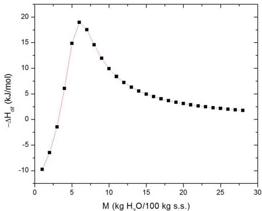
Figura A2. Entalpía diferencial de las microcápsulas
