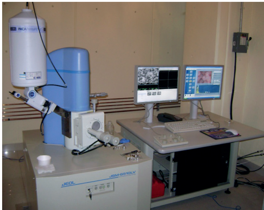
FIGURA 1. Microscopio electrónico de barrido – Espectroscopía por dispersión de energía de rayos-X para análisis elemental y mapeo químico.
